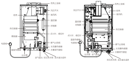
(内部结构图)
